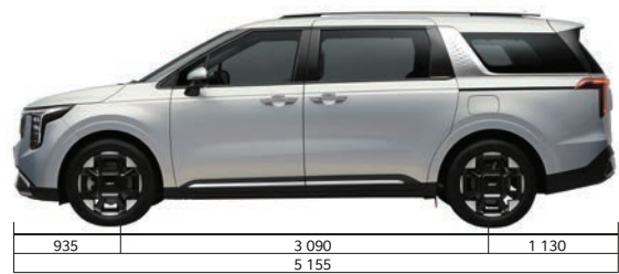
Размеры (мм), 18" колеса
